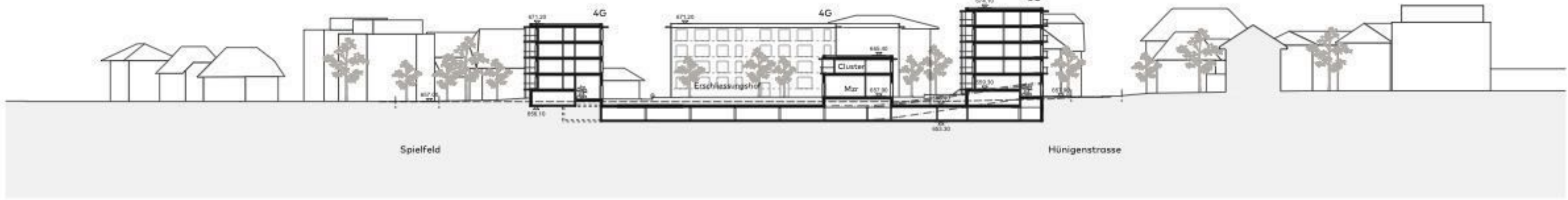
Schnitt C-C 1:500
