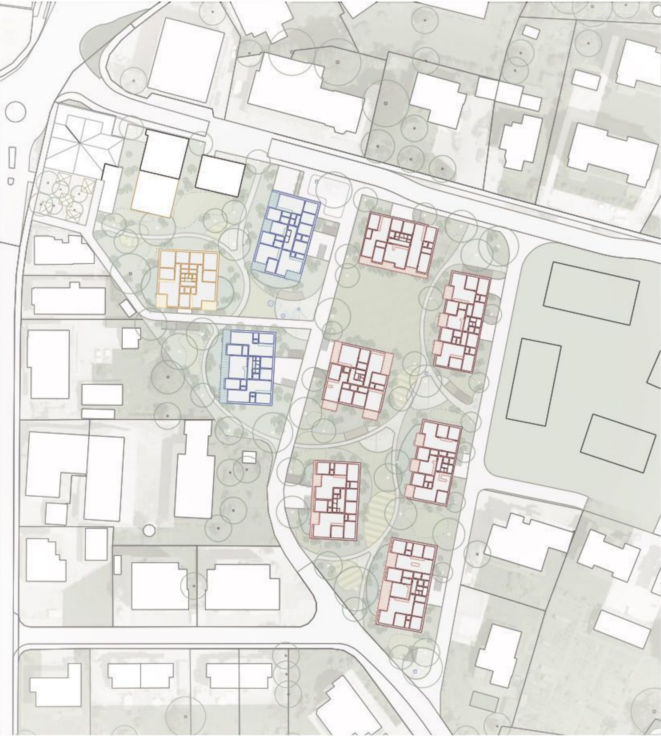
Grundriss Regelgeschoss - 1:500
