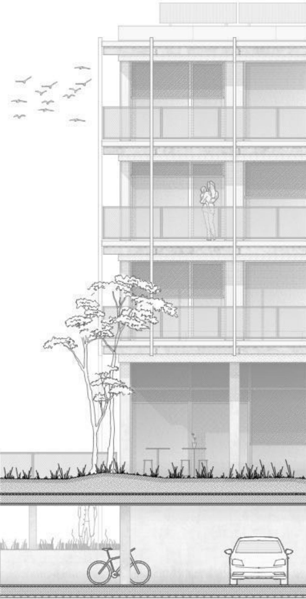
Ansicht Baufeld B 1:50
