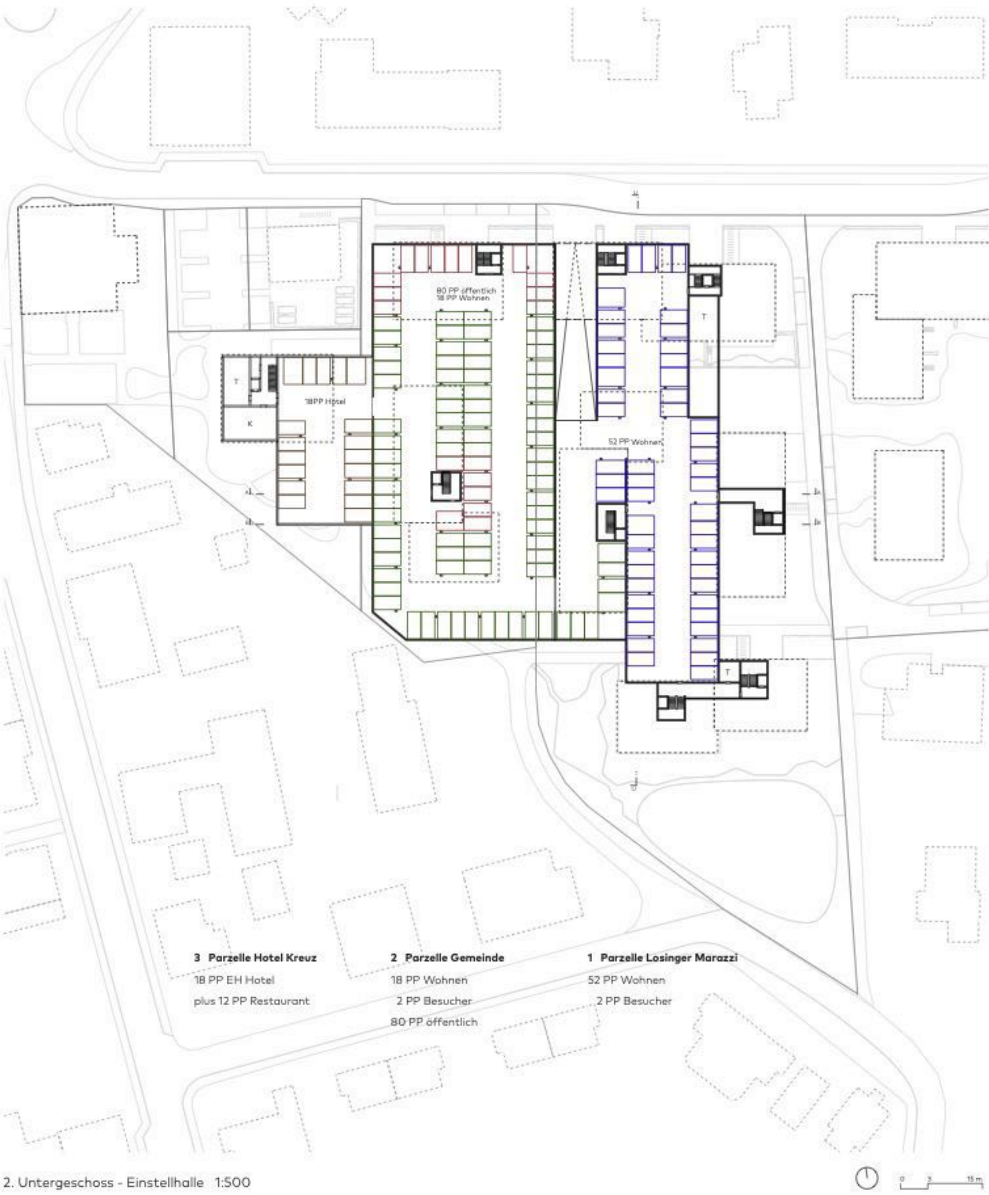
2. Untergeschoss - Einstellhalle 1:500
