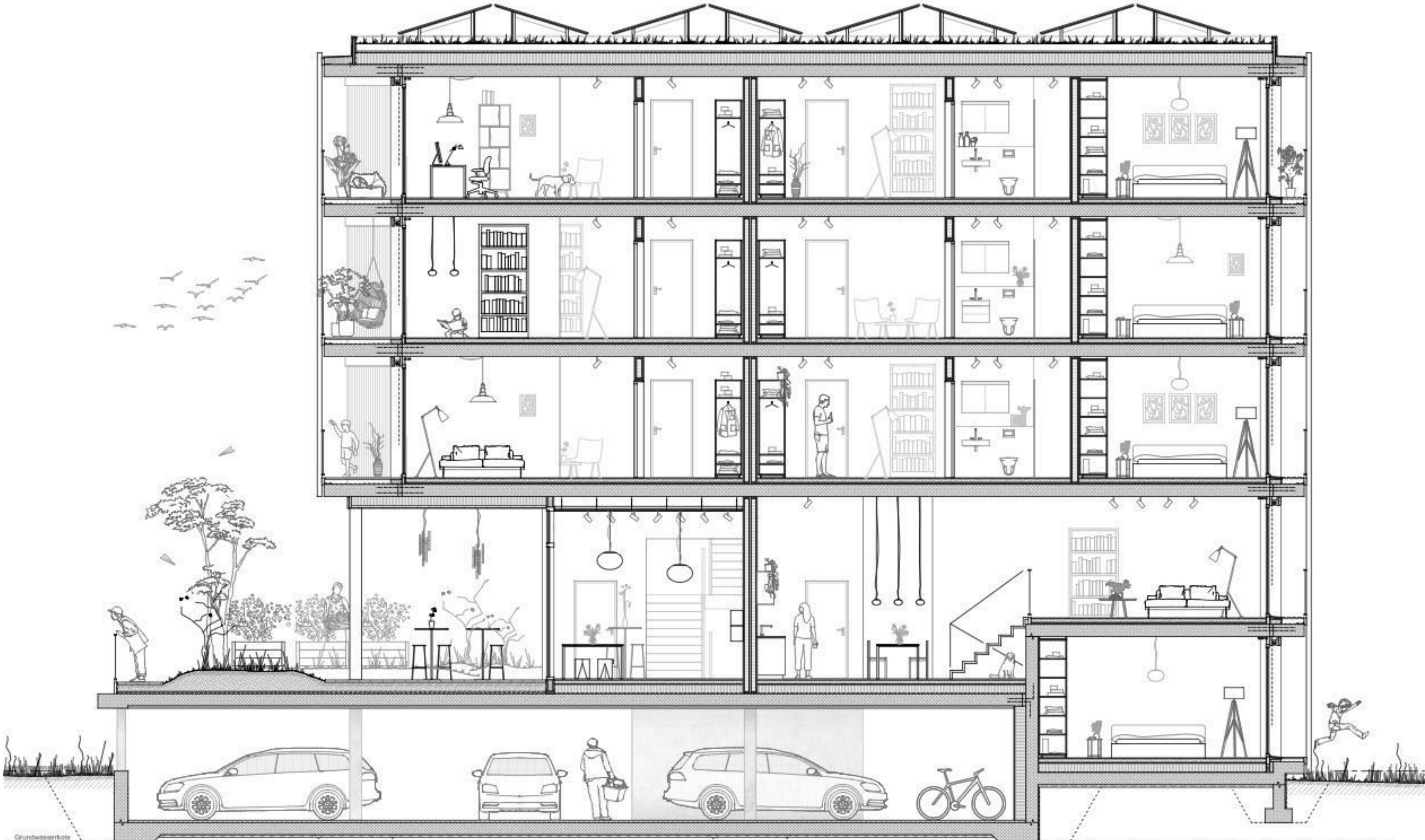
Detailschnitt Baufeld B 1:50
